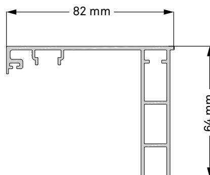
Profilo coprifilo lungo Long casing profile
