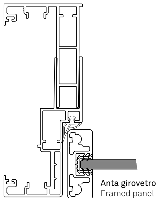
Assieme anta + telaio Door + frame assembly
