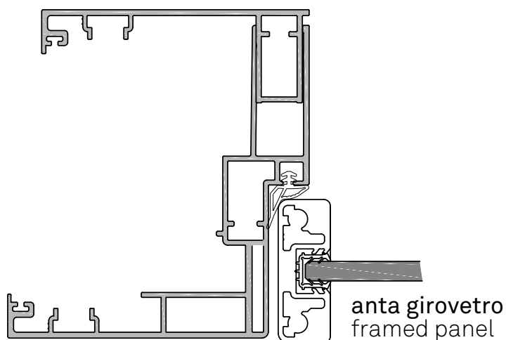
Assieme anta + telaio Door + frame assembly
