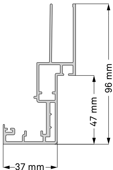
Profilo di prolunga ad H H extension profile
