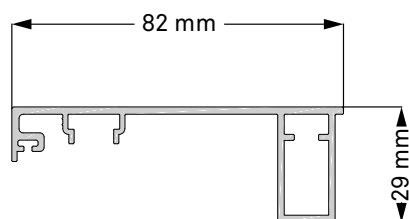
Profilo coprifilo corto Short casing profile
