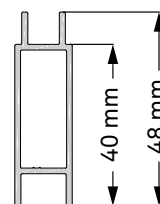
Profilo di prolunga ad H H extension profile
