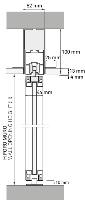
BINARIO 1 VIA PER CONTROSOFFITTO 1 WAY TRACK FOR FALSE CEILING
