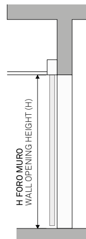
PER CONTROSOFFITTO AT THE FALSE CEILING
