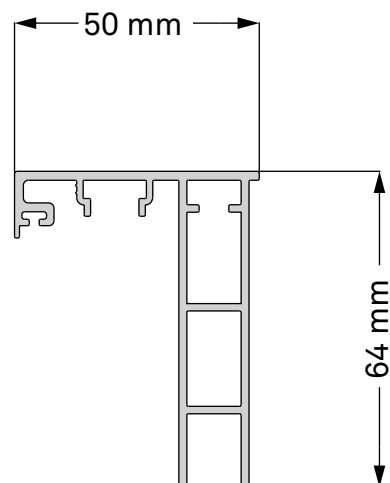
Profilo coprifilo Casing profile
